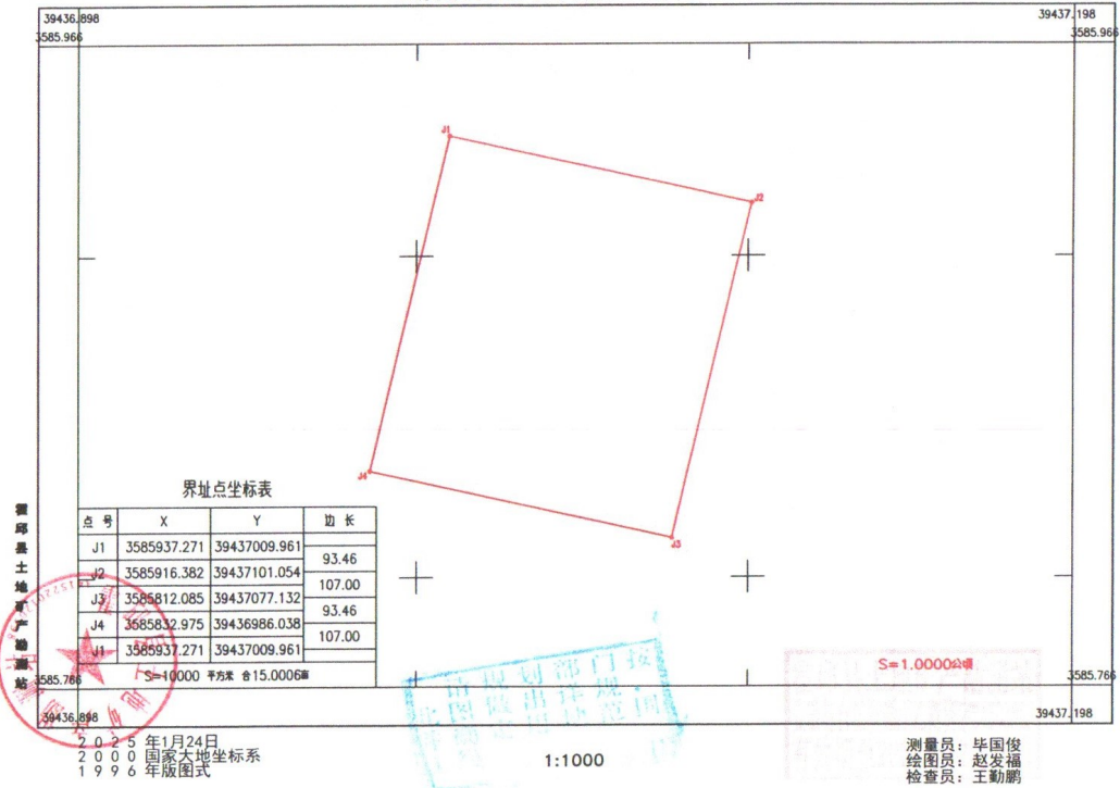
新店镇收储地块勘测定界图
