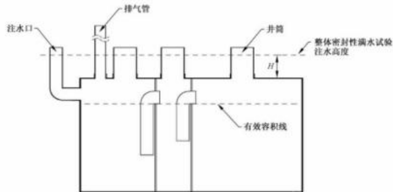
图 B.1 三格化粪池密封试验示意图
