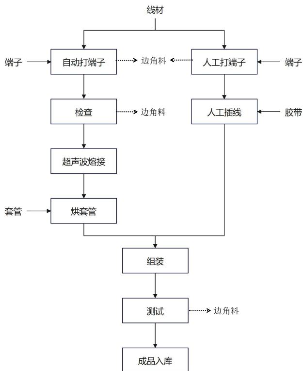
图 2.4 汽车组合线束生产工艺
