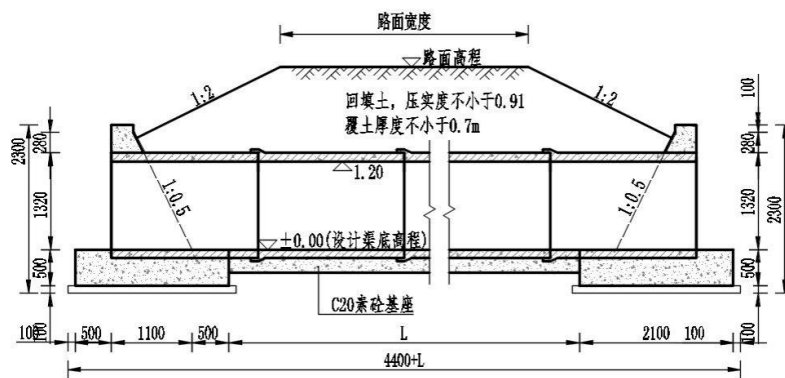
图 2-5 \Phi 1200\text{mm} 过路涵横断面结构图
