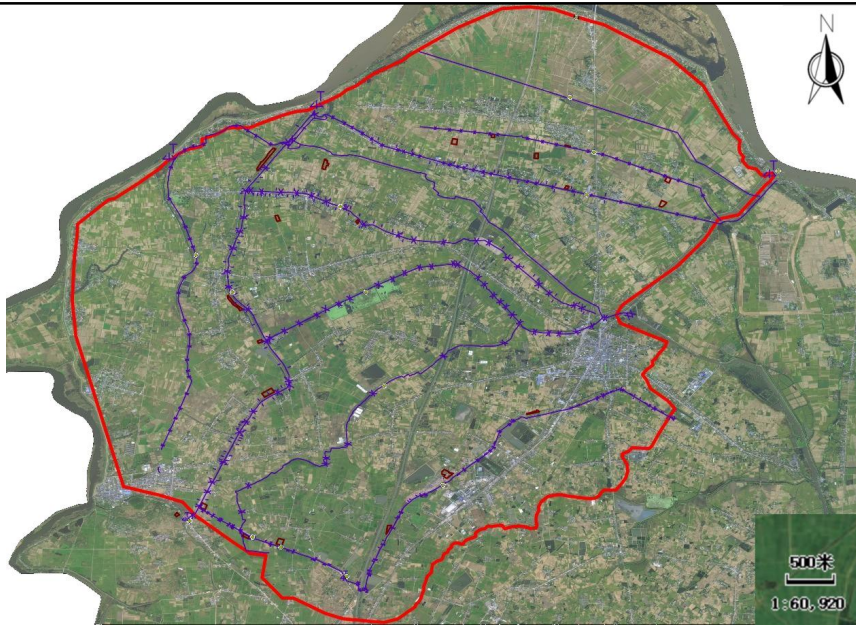
图2-12 临时堆土场分布图
