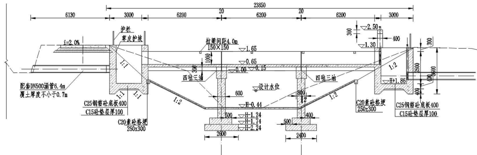
图2-7 渡槽典型设计图
