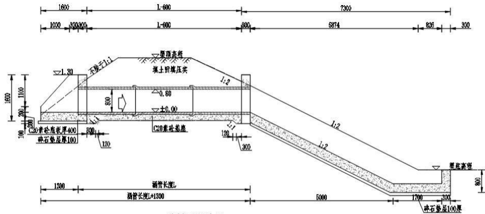
纵剖面设计图 1:50
