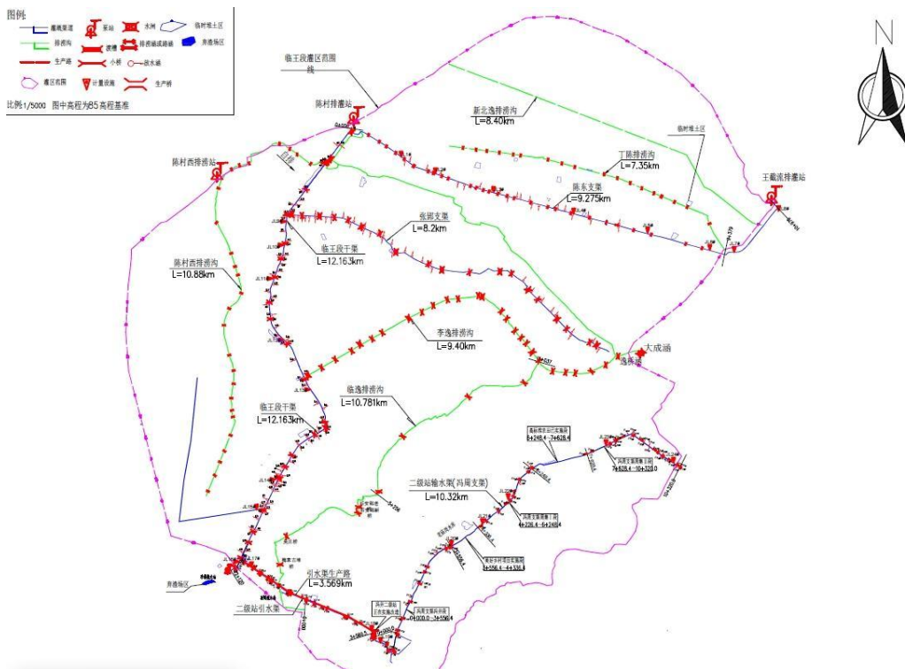
图2-9 工程总体布置图
