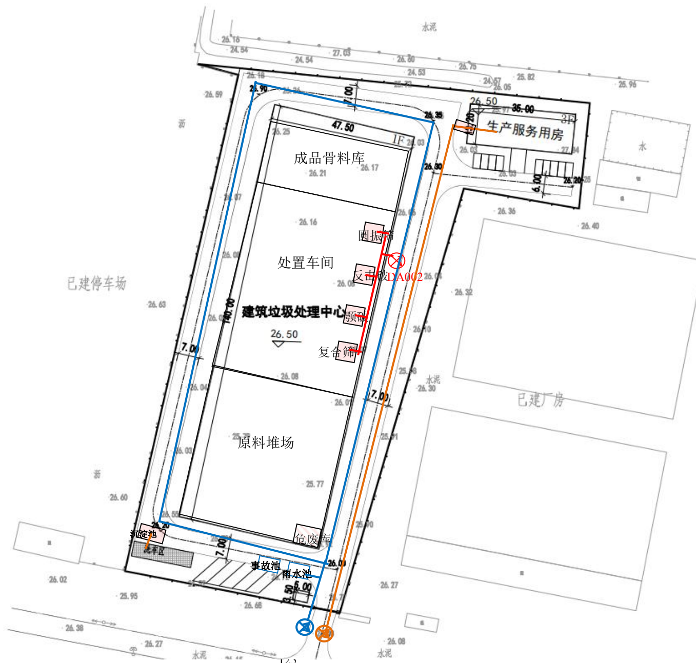
附图 4-2 资源化利用工程平面布置图
