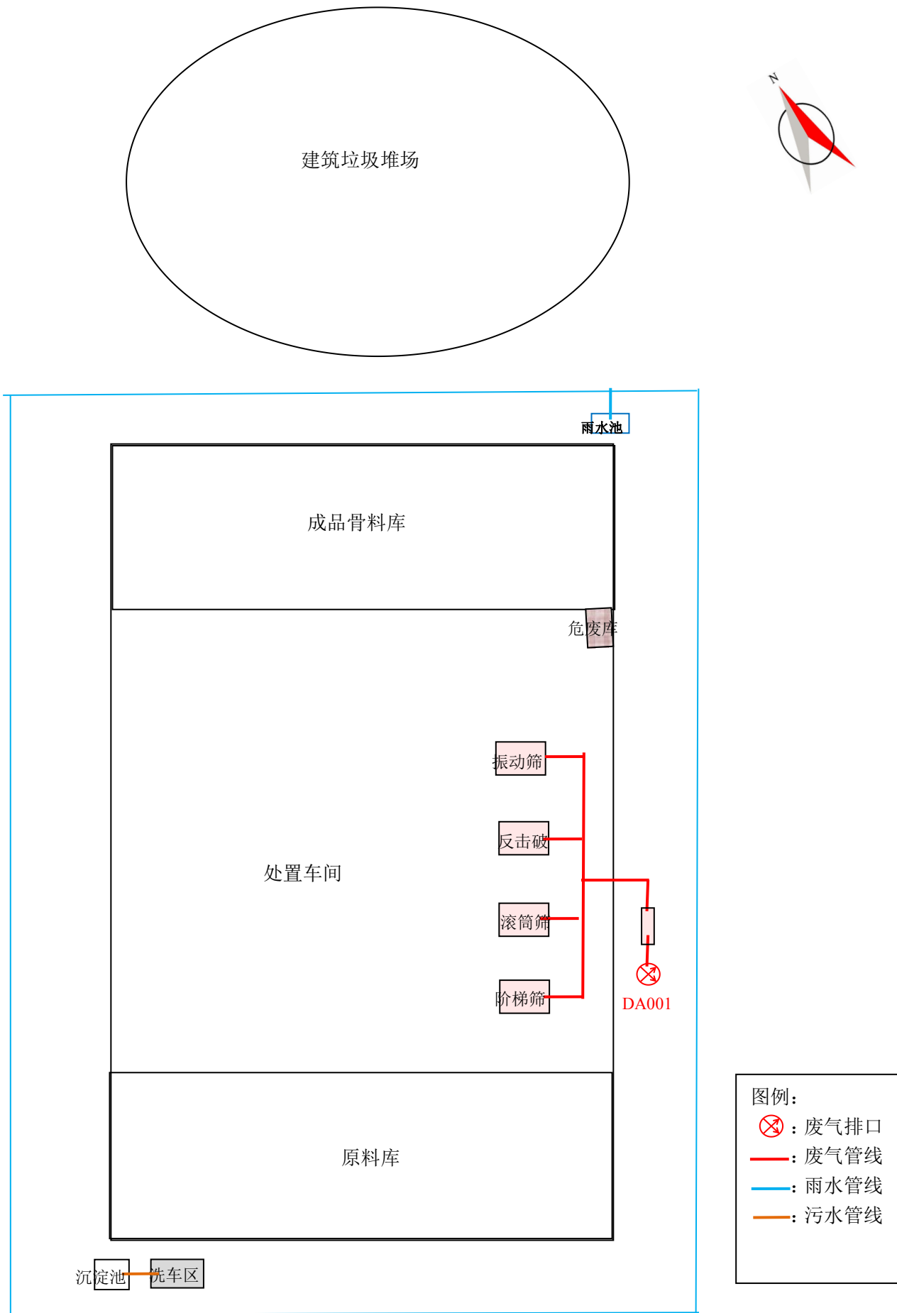
附图 4-1 环境综合整治工程平面布置图
